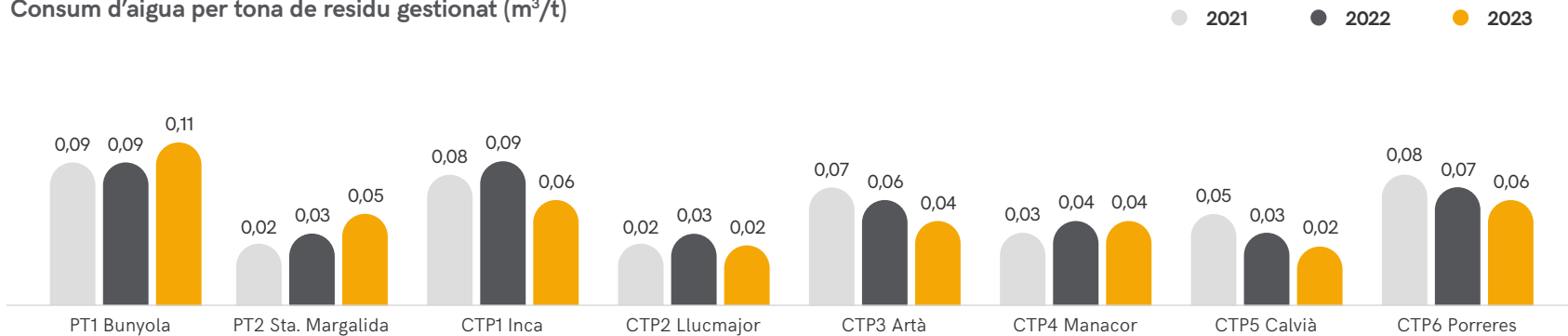
Consum d'aigua per tona de residu gestionat (m 3 /t)
